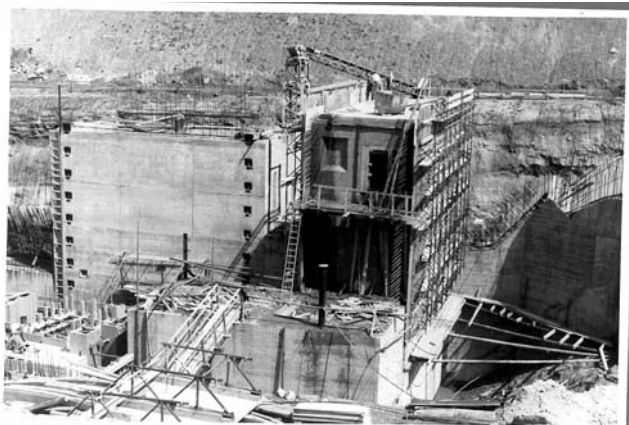
Schleusenoberhaupt 1969
